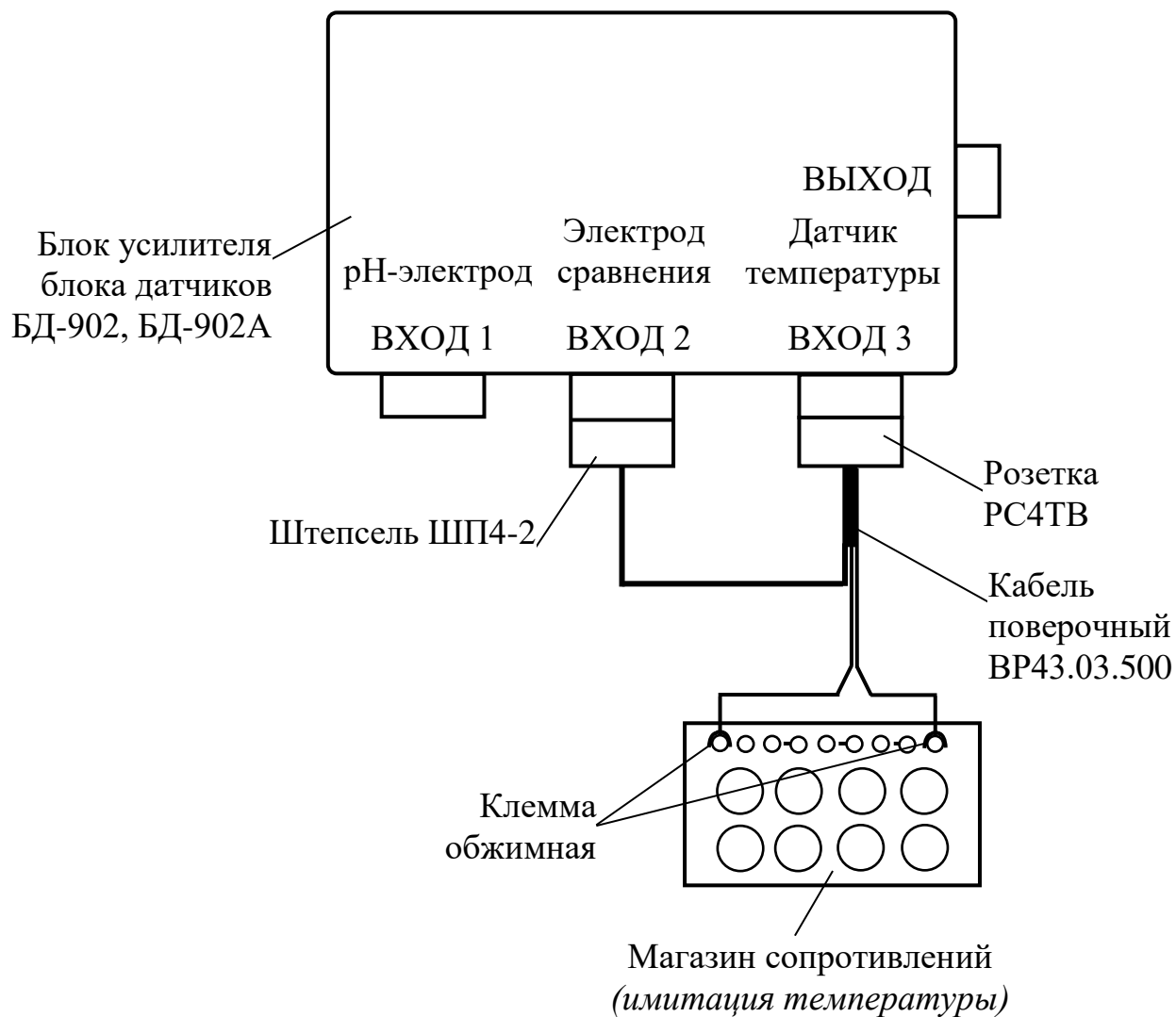
Рисунок Д.3 – Схема подключения кабеля поверочного BP43.03.500
