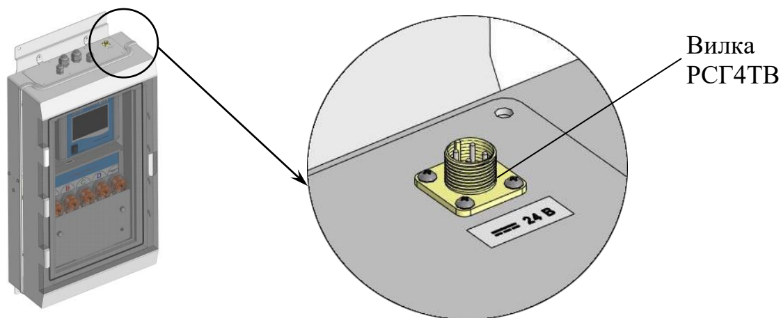
Рисунок 11.1 – Расположение разъема « \text{---} 24 В» на модуле измерительном
