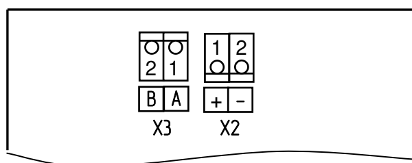
в – схема расположения разъемов на плате блока управления клапанами
