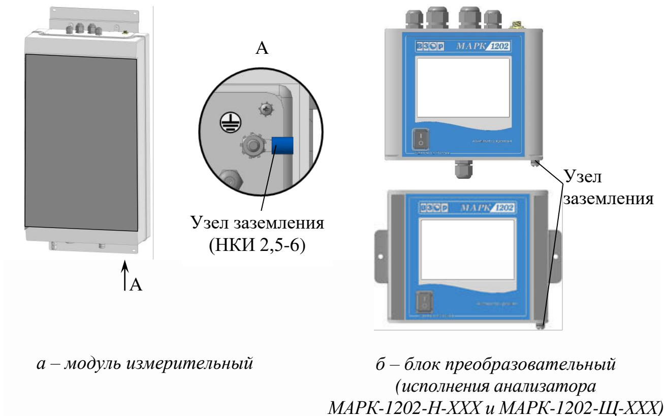
Рисунок 10.1 – Расположение узлов заземления
