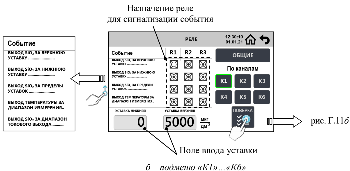
Рисунок Г.12 – Экраны меню «РЕЛЕ»
