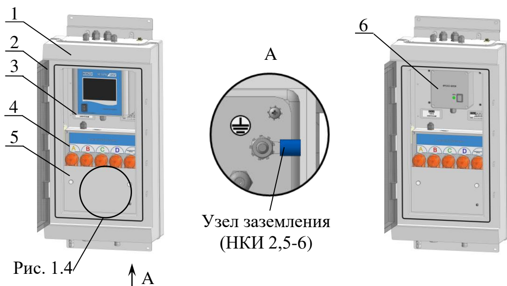
а – исполнение BP79.01.000 (BP79.01.000-01)
