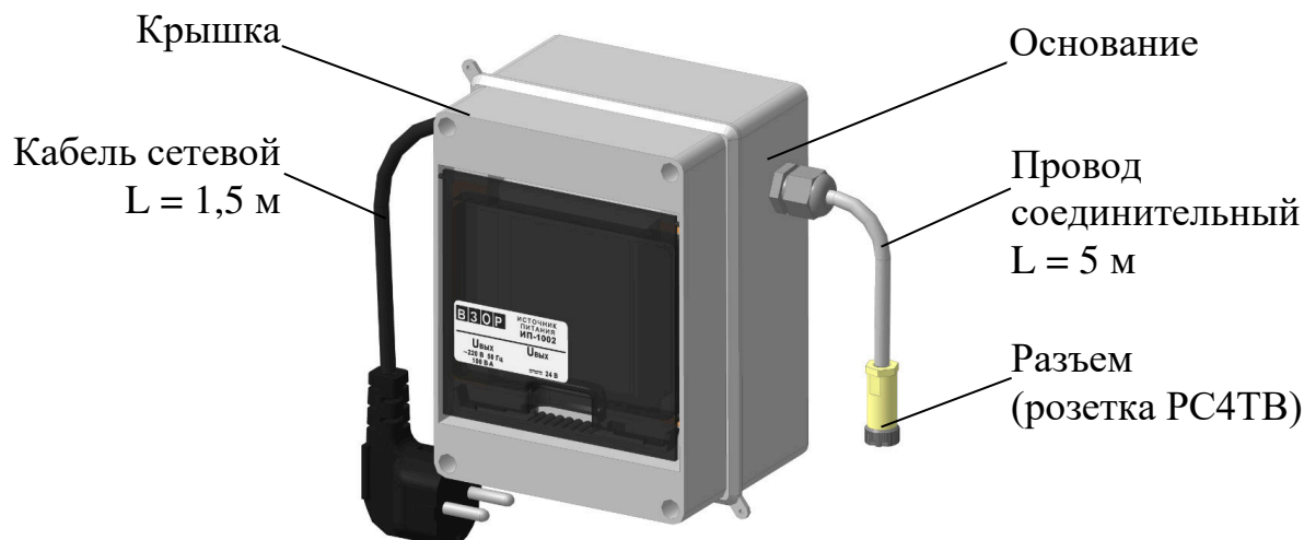
Рисунок 1.10 – Источник питания ИИ-1002 BP49.04.000
