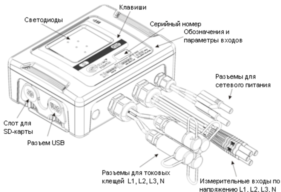
Рис.1 Анализатор качества электрической энергии PQM-700. Общий вид.
