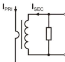
Рис.16 Жёсткие клещи с выходом по напряжению.
