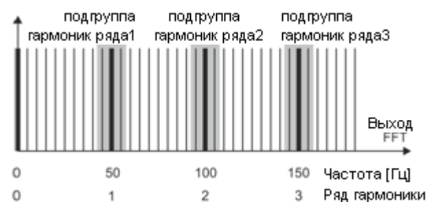
Рис.15 Определение подгрупп гармоник (сеть 50 Гц)
