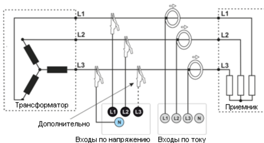
Рис.8 Схема подключения – трёхфазная сеть «звезда» с изолированной нейтрью.
