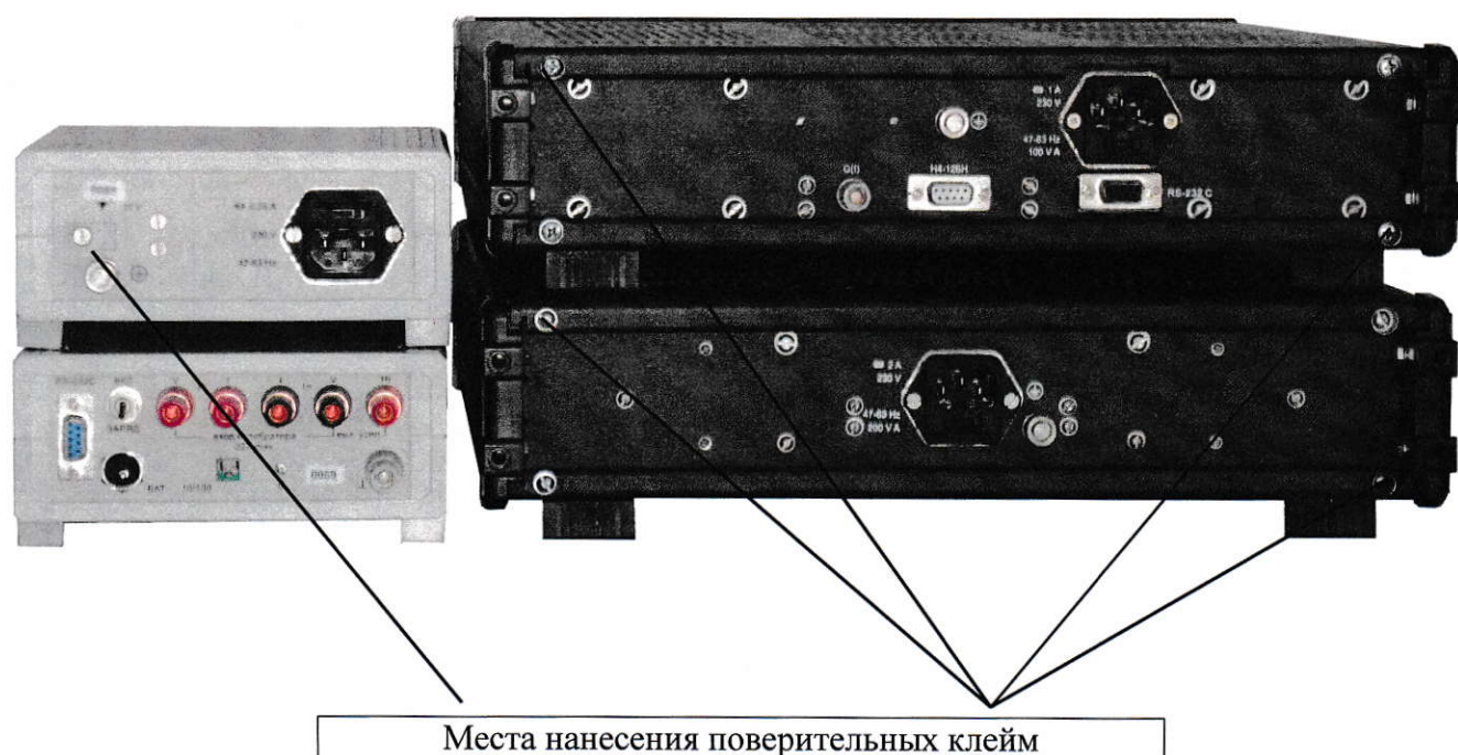
Рисунок 1 - Общий вид калибратора-вольтметра универсального Н4-12
