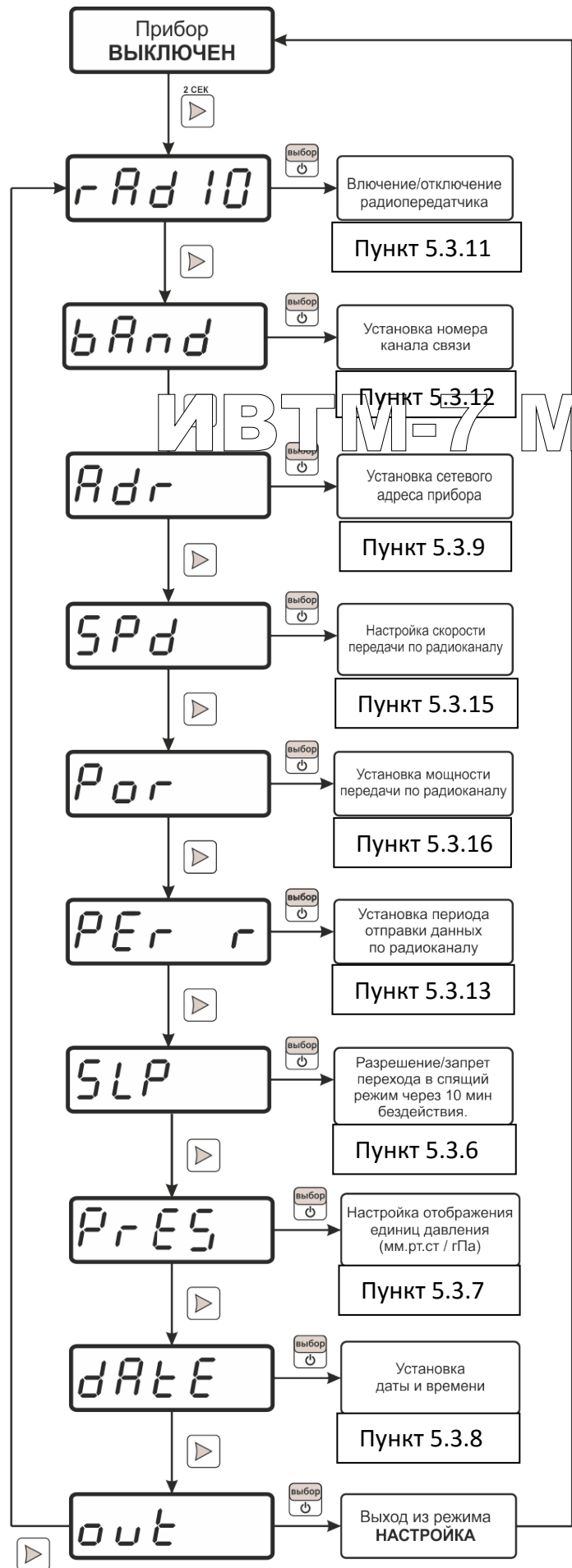
Рисунок 5.21 Схема режима НАСТРОЙКА ИВТМ-7 М 4(-Д)
