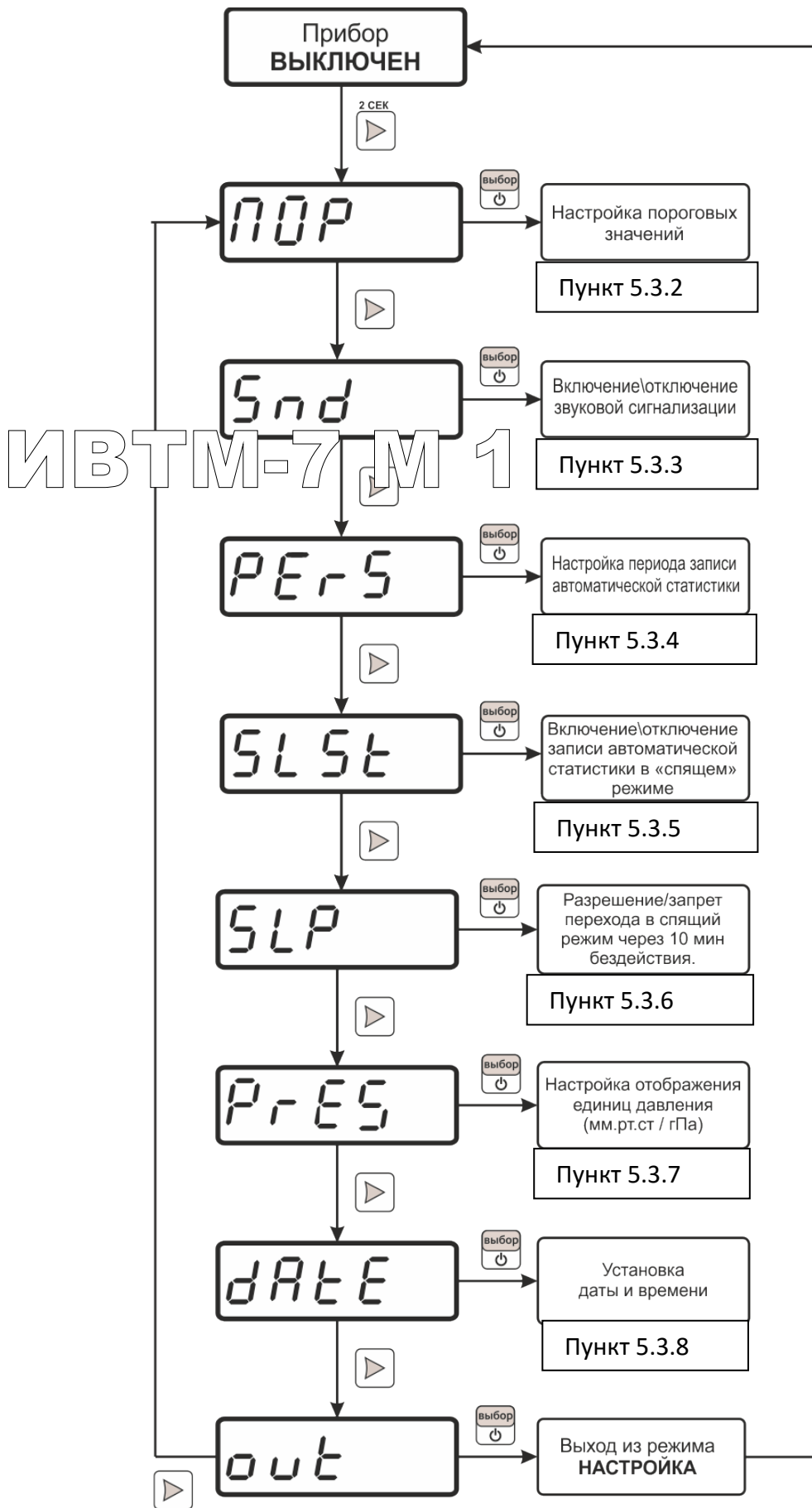
Рисунок 5.18 Схема режима НАСТРОЙКА ИВТМ-7 М 1
