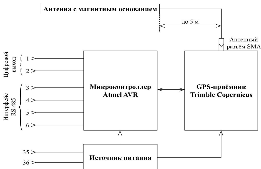
Рис. 2.2. Структурная схема Модуля МКВ-02Ц
