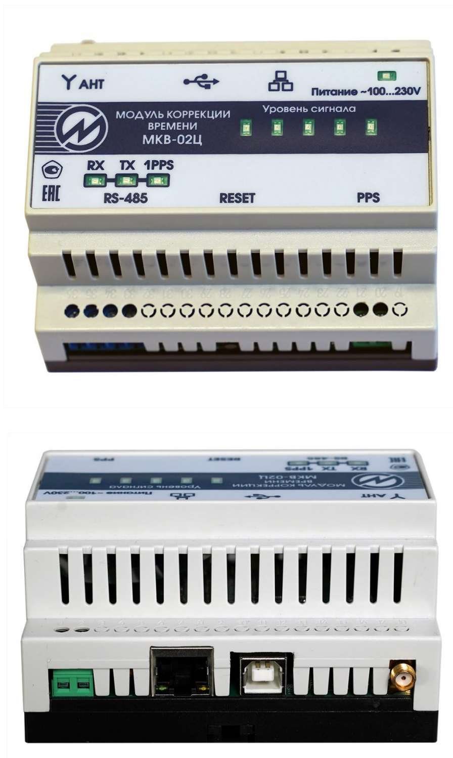
Рис. 3.1. Расположение соединителей, клемм и индикаторов Модуля MKB-02Ц
