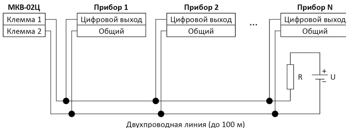
Рис. А.1. Схема подключения Модуля МКВ-02Ц к Приборам
