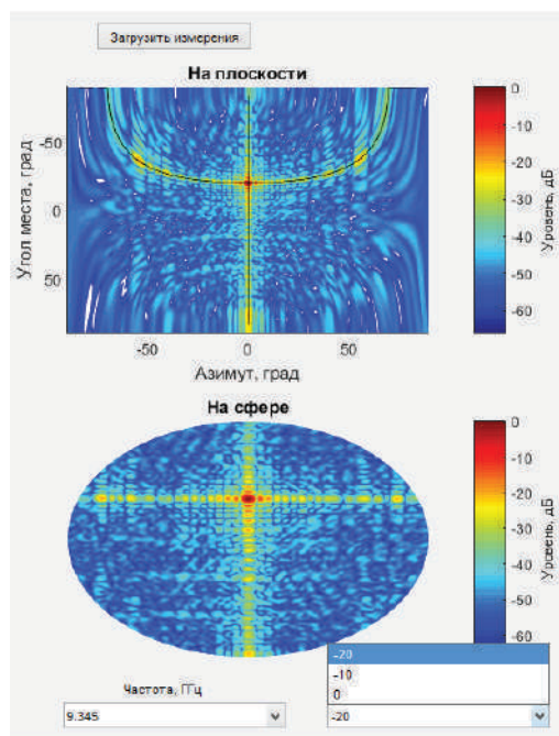
АФР, измеренное в ближней зоне
