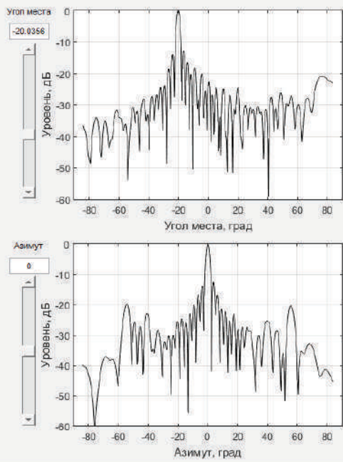
АФР, восстановленное на полотно АФР с отказавшим элементом
