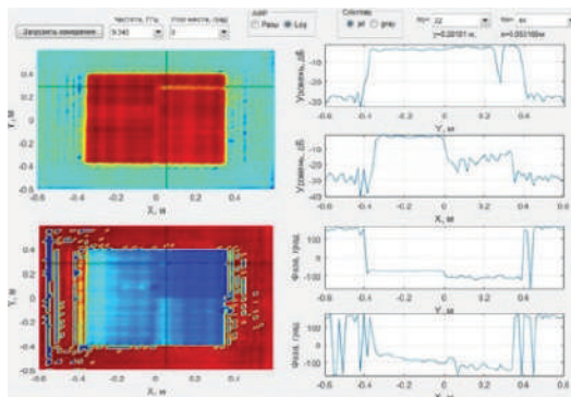
АФР, восстановленное на полотно АФР с отказавшим элементом
